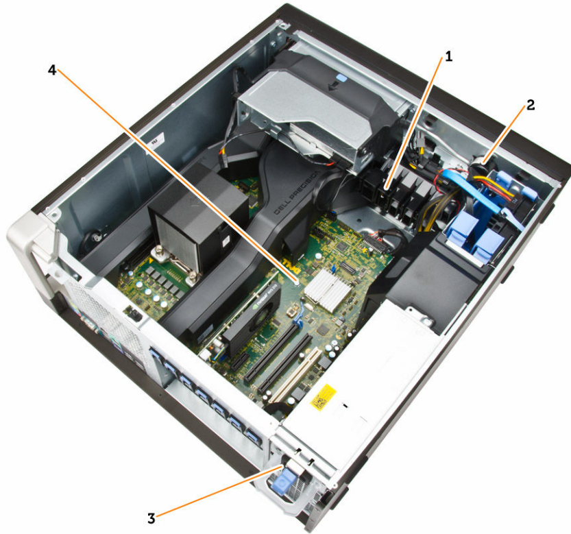
그림 3. T5810 컴퓨터 내부
