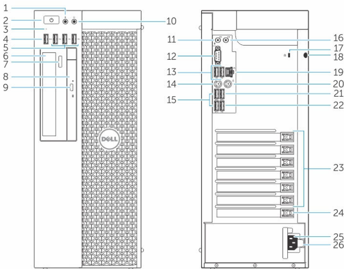
그림 1. T5810 컴퓨터의 전면 및 후면 모습
