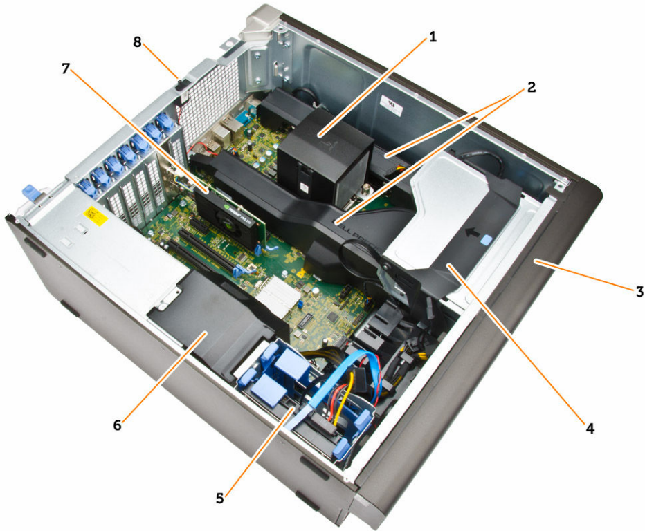
그림 2 . T5810 컴퓨터 내부
